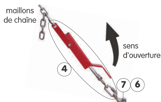
Figure 9 : Câblerie en tension : Tendeur rapide fermé
