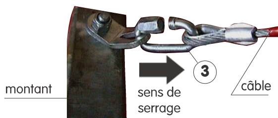
Figure 6 - Montage maillon rapide (3) / tendeur à lanterne (8)
