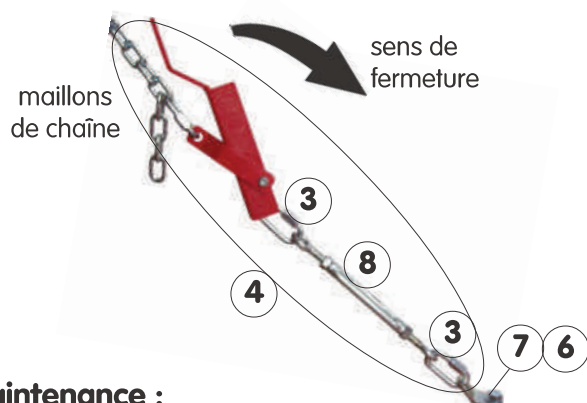
Figure 8 - Câblerie détendue : Tendeur rapide ouvert
