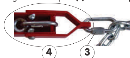
Figure 7 - Montage maillon rapide (3) / tendeur rapide (4)
